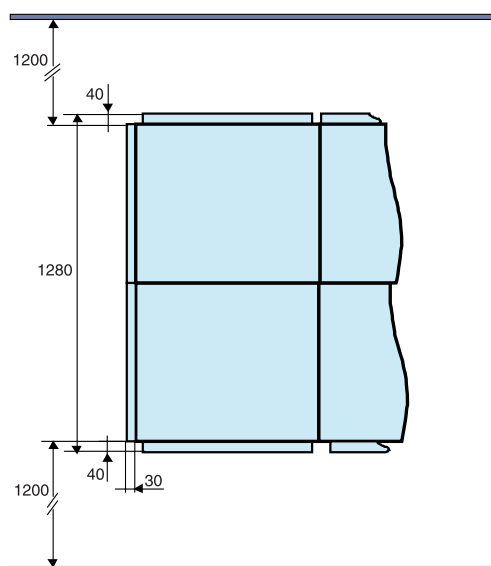
Ячейка с задним присоединением глубиной 1200 мм: минимальное пространство спереди и сзади
