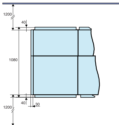
Ячейка с задним присоединением глубиной 1000 мм: минимальное пространство спереди и сзади
