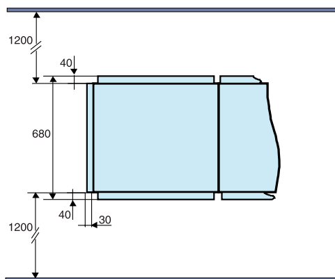
Ячейка с задним присоединением глубиной 600 мм: минимальное пространство спереди и сзади
