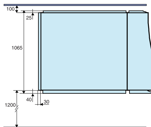
Ячейка с передним присоединением NW40b/50/63/3 полюса: минимальное пространство спереди и сзади
