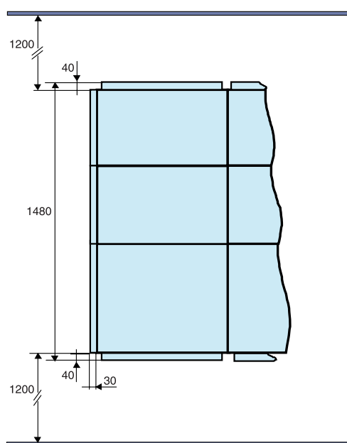
Ячейка с задним присоединением глубиной 1400 мм: минимальное пространство спереди и сзади
