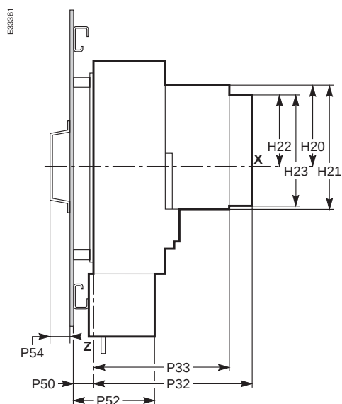
Стационарный аппарат
