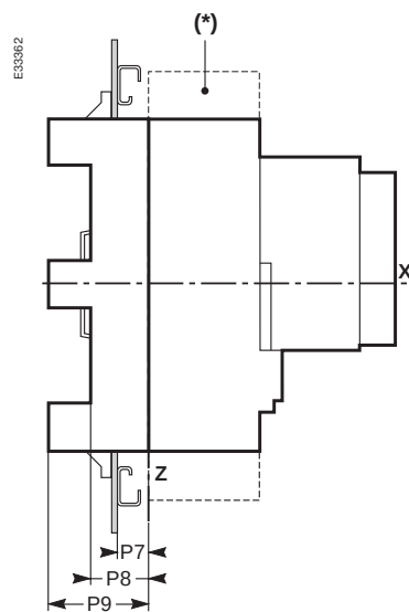
Выдвижной аппарат
