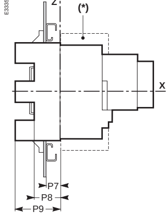
Выдвижной аппарат
