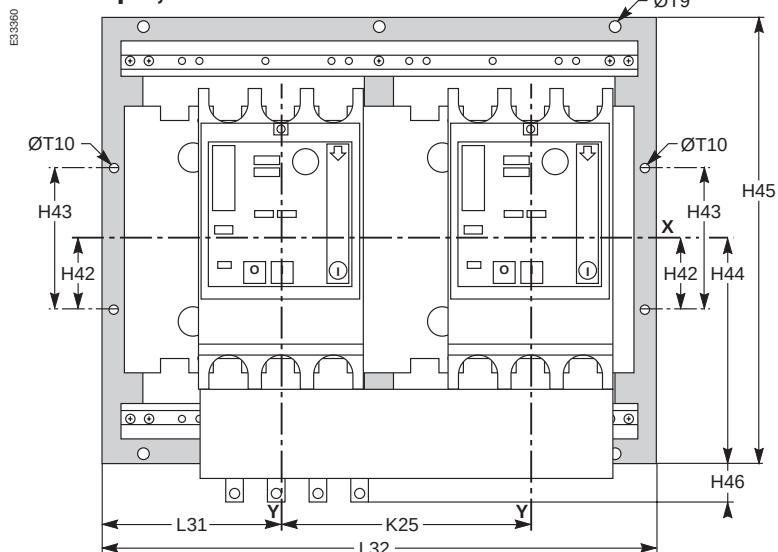
Стационарный аппарат
