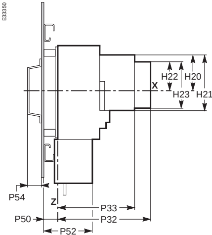
Стационарный аппарат
