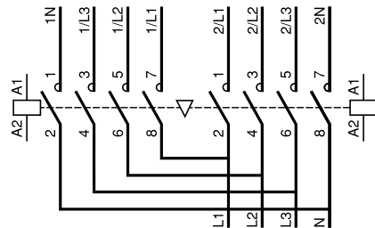
Контакторы автоматического ввода резерва для распределительных сетей, горизонтального крепления LC2-F 2 x LC1-F
