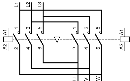
Реверсивные контакторы для управления электродвигателями, горизонтального крепления LC2-F 2 x LC1-F
