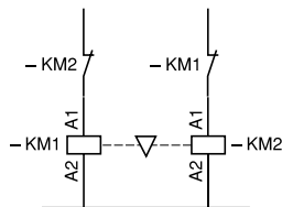
Электрическая блокировка реверсивных контакторов, оснащенных механической блокировкой без встроенных электрических контактов LA9-F●●●
